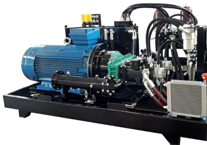
Centrale per trituratore circuito chiuso (315 kW)
