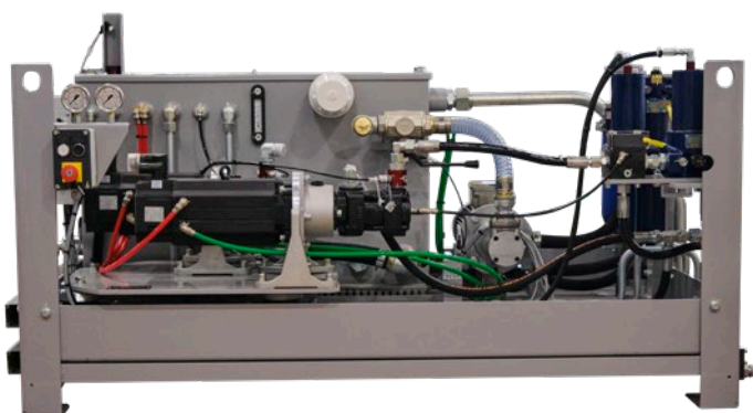
Centrale idraulica per punzonatrice con servo pompa
